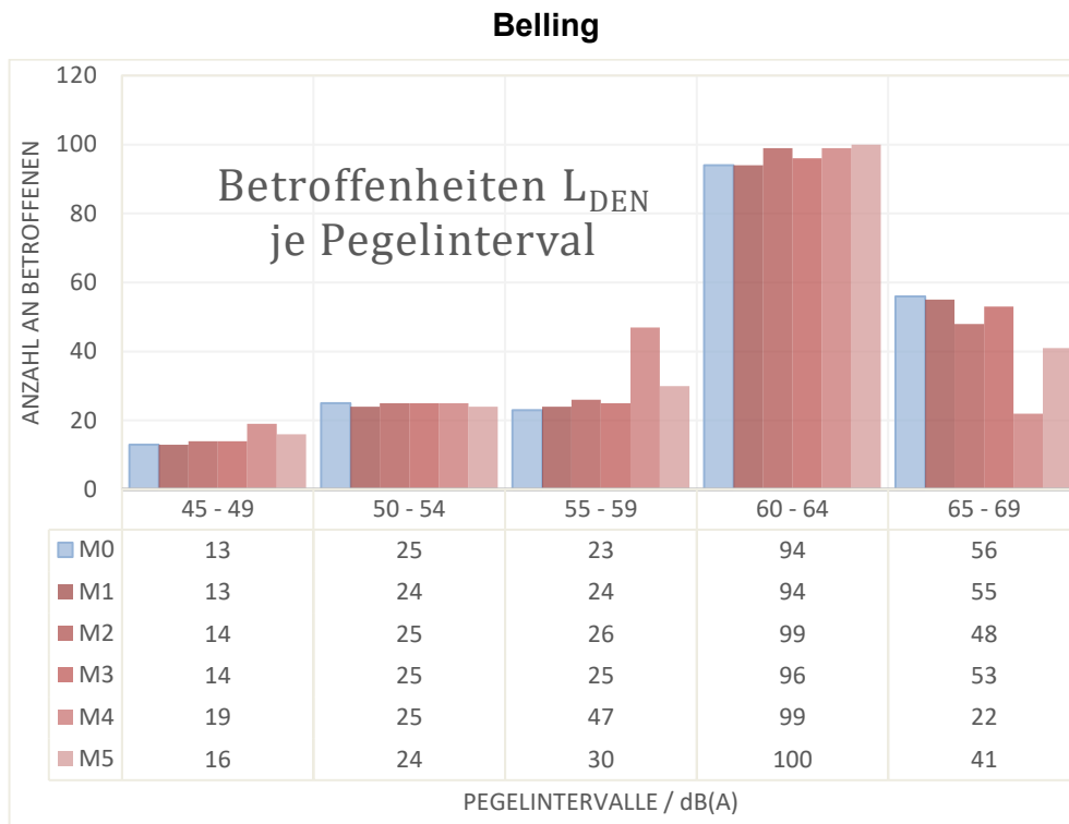
Abbildung 11: Angabe der Betroffenheiten je Pegelintervall im Zeitraum L_{DEN} für Belling. Die Betroffenheiten sind hierbei als Balken, sowie in absoluten Zahlen darunter gegeben. (Beispiel: Die Bestand-Situation weist im Pegelintervall 50-54 dB(A), 25 Betroffene auf (blauer Balken)).
