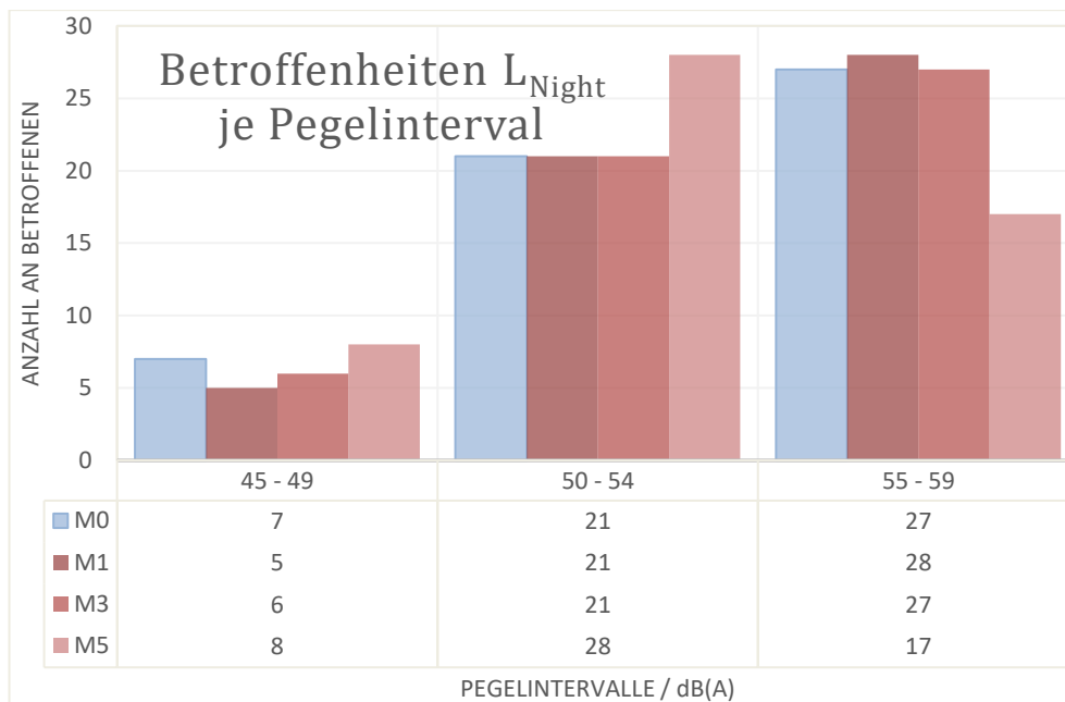
Abbildung 8: Angabe der Betroffenheiten je Pegelintervall im Zeitraum L_{Night} für Wilhelmsthal/Sandförde. Die Betroffenheiten sind hierbei als Balken, sowie in absoluten Zahlen darunter gegeben. (Beispiel: Die Bestand-Situation weist im Pegelintervall 45-49 dB(A) 7 Betroffene auf (blauer Balken)). Nachts ist Maßnahme M3 = Maßnahme M2 und Maßnahme M5 = Maßnahme M4
