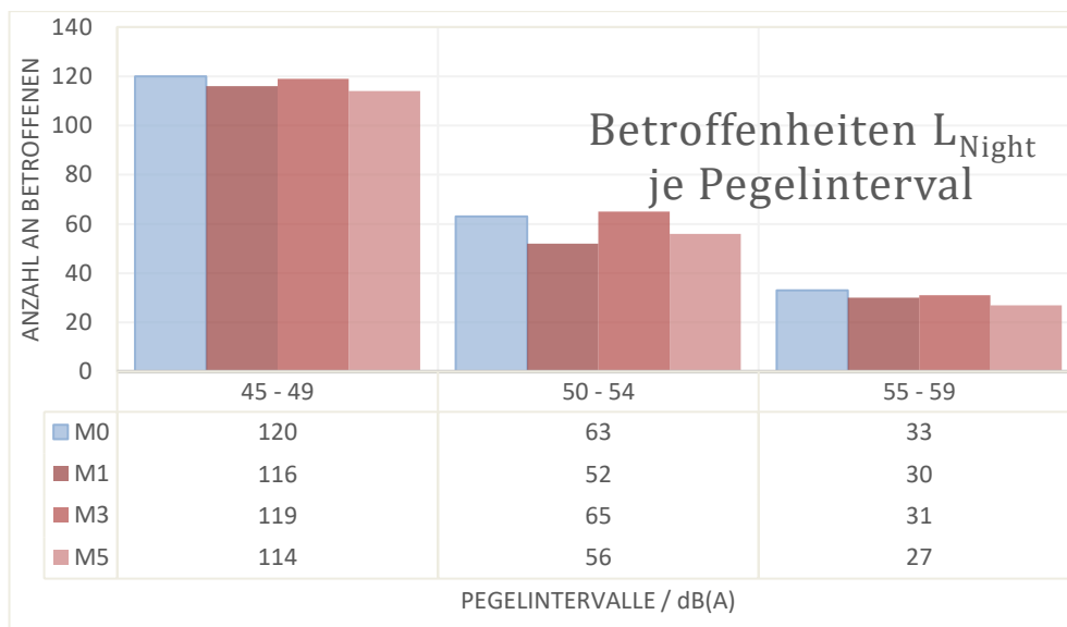
Abbildung 20: Angabe der Betroffenheiten je Pegelintervall im Zeitraum L_{Night} für Rollwitz. Die Betroffenheiten sind hierbei als Balken, sowie in absoluten Zahlen darunter gegeben. (Beispiel: Die Bestand-Situation weist im Pegelintervall 45-49 dB(A), 120 Betroffene auf (blauer Balken)). Nachts ist Maßnahme M3 = Maßnahme M2 und Maßnahme M5 = Maßnahme M4
