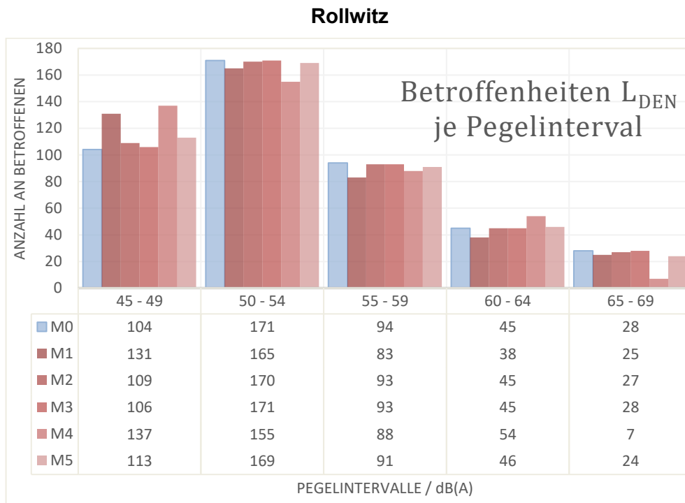
Abbildung 19: Angabe der Betroffenheiten je Pegelintervall im Zeitraum L_{DEN} für Rollwitz. Die Betroffenheiten sind hierbei als Balken, sowie in absoluten Zahlen darunter gegeben. (Beispiel: Die Bestand-Situation weist im Pegelintervall 50-54 dB(A), 171 Betroffene auf (blauer Balken)).
