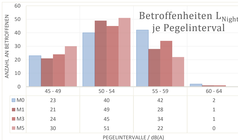
Abbildung 18: Angabe der Betroffenheiten je Pegelintervall im Zeitraum L_{Night} für Polzow. Die Betroffenheiten sind hierbei als Balken, sowie in absoluten Zahlen darunter gegeben. (Beispiel: Die Bestand-Situation weist im Pegelintervall 45-49 dB(A), 23 Betroffene auf (blauer Balken)). Nachts ist Maßnahme M3 = Maßnahme M2 und Maßnahme M5 = Maßnahme M4
