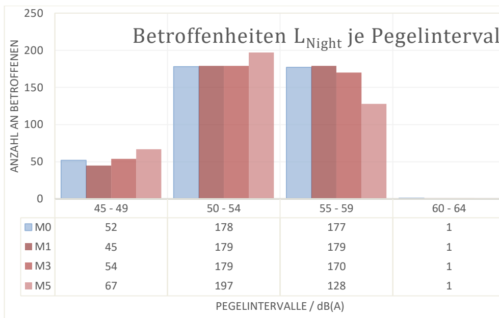
Abbildung 14: Angabe der Betroffenheiten je Pegelintervall im Zeitraum L_{Night} für Jatznick. Die Betroffenheiten sind hierbei als Balken, sowie in absoluten Zahlen darunter gegeben. (Beispiel: Die Bestand-Situation weist im Pegelintervall 45-49 dB(A), 52 Betroffene auf (blauer Balken)). Nachts ist Maßnahme M3 = Maßnahme M2 und Maßnahme M5 = Maßnahme M4
