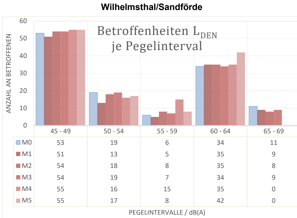
Abbildung 7: Angabe der Betroffenheiten je Pegelintervall im Zeitraum L_{DEN} für Wilhelmsthal/Sandförde. Die Betroffenheiten sind hierbei als Balken, sowie in absoluten Zahlen darunter gegeben. (Beispiel: Die Bestand-Situation weist im Pegelintervall 50-54 dB(A), 19 Betroffene auf (blauer Balken)).
