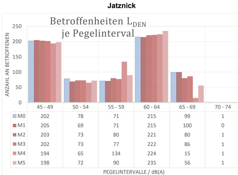
Abbildung 13: Angabe der Betroffenheiten je Pegelintervall im Zeitraum L_{DEN} für Jatznick. Die Betroffenheiten sind hierbei als Balken, sowie in absoluten Zahlen darunter gegeben. (Beispiel: Die Bestand-Situation weist im Pegelintervall 50-54 dB(A), 78 Betroffene auf (blauer Balken)).
