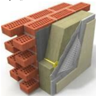
Isolierung
